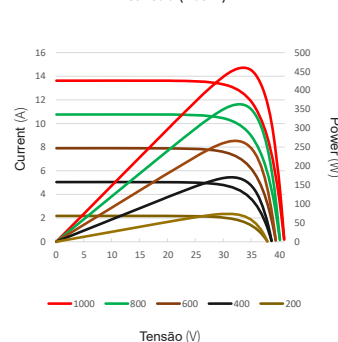
Curvas de corrente-tensão e potência-tensão (465W)
