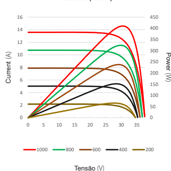
Curvas de corrente-tensão e potência-tensão (405W)
