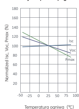
Charakterystyka zmiany mocy w funkcji temperatury ognia
