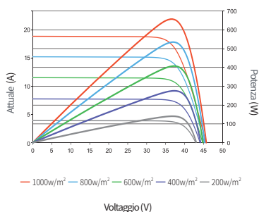
Curve corrente-tensione e potenza-tensione (665W)
