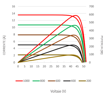
Curvas de corriente-voltaje y potencia-voltaje (580W)
