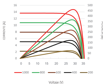
Curvas de corriente-voltaje y potencia-voltaje (470W)
