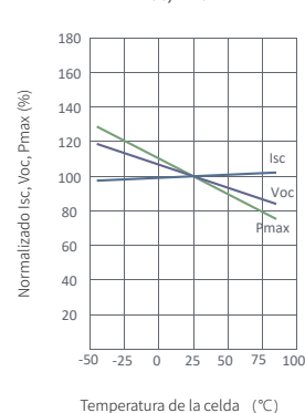
Dependencia de temperatura de I_{sc} , V_{oc} , P_{max}
