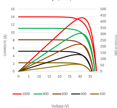
Curvas de corriente-voltaje y potencia-voltaje (430W)
