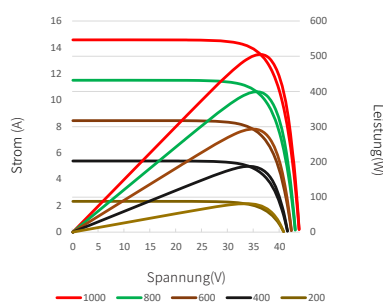
Strom-Spannungs- und Leistungs-Spannungs-Diagramme(500W)
