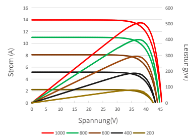
Strom-Spannungs- und Leistungs-Spannungs-Diagramme(495W)
