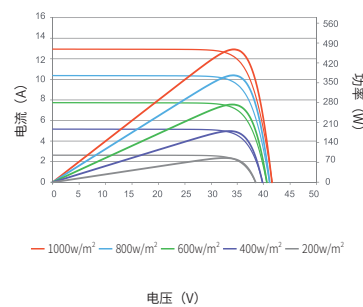
电流 - 电压 & 功率 - 电压曲线图 (460W)
