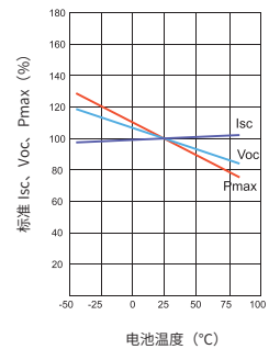
I_{sc} , V_{oc} , P_{max} 的温度曲线
