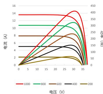
电流 - 电压 & 功率 - 电压曲线图 (410W)
