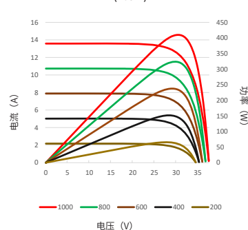
电流 - 电压 & 功率 - 电压曲线图 (405W)
